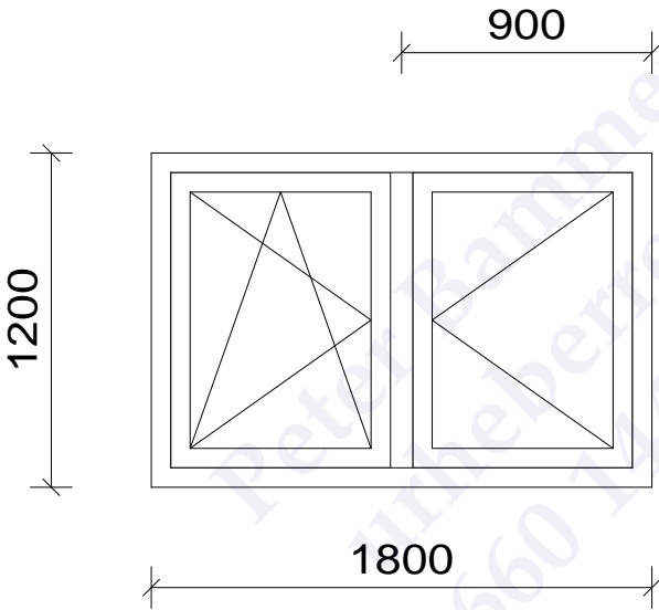
Fenster, einfach 2 Flügel, 74975
